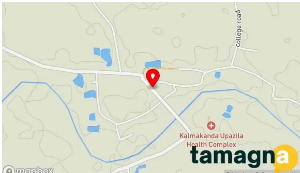
Dagre map
