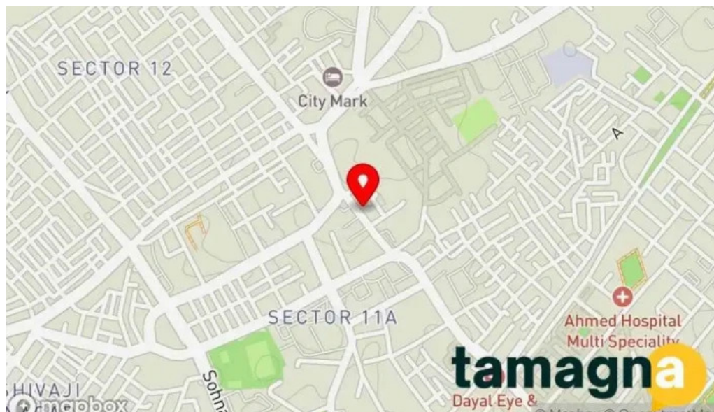
Sai om computers map
